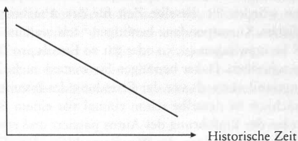
Abb. 2: Für die Ausführung einer bestimmten Handlung (etwa das Zurücklegen einer zehn Kilometer langen Strecke, die Vervielfältigung eines Buches oder die Beantwortung von zehn Nachrichten) benötigte Zeitressourcen im Zeitalter der technischen Beschleunigung (vgl. Abb. 1.).
