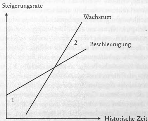
Abb. 3: »Freizeit« (1) bzw. »Zeitknappheit« (2) sind Folgen des Verhältnisses von Wachstumsraten und Beschleunigungsraten. (1) bildet ein abnehmendes und (2) ein zunehmendes Lebenstempo ab. Sind beide Raten identisch (also an der Stelle, an der sie sich kreuzen), dann bleibt das Lebenstempo trotz technischer Beschleunigung unverändert. In der Beschleunigungsgesellschaft übertreffen Wachstumsraten Beschleunigungsraten auf systematische Weise (2)
