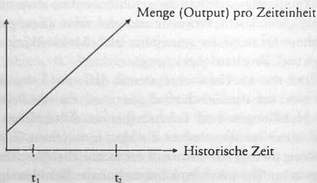
Abb. 1: Technische Beschleunigung als Mengenzunahme pro Zeiteinheit. t_1 und t_2 können im Fall der Transportgeschwindigkeit in Stundenkilometern für 1800 und 1950 oder im Fall der Betriebsgeschwindigkeit von Computern für 1960 und 2000 stehen.
